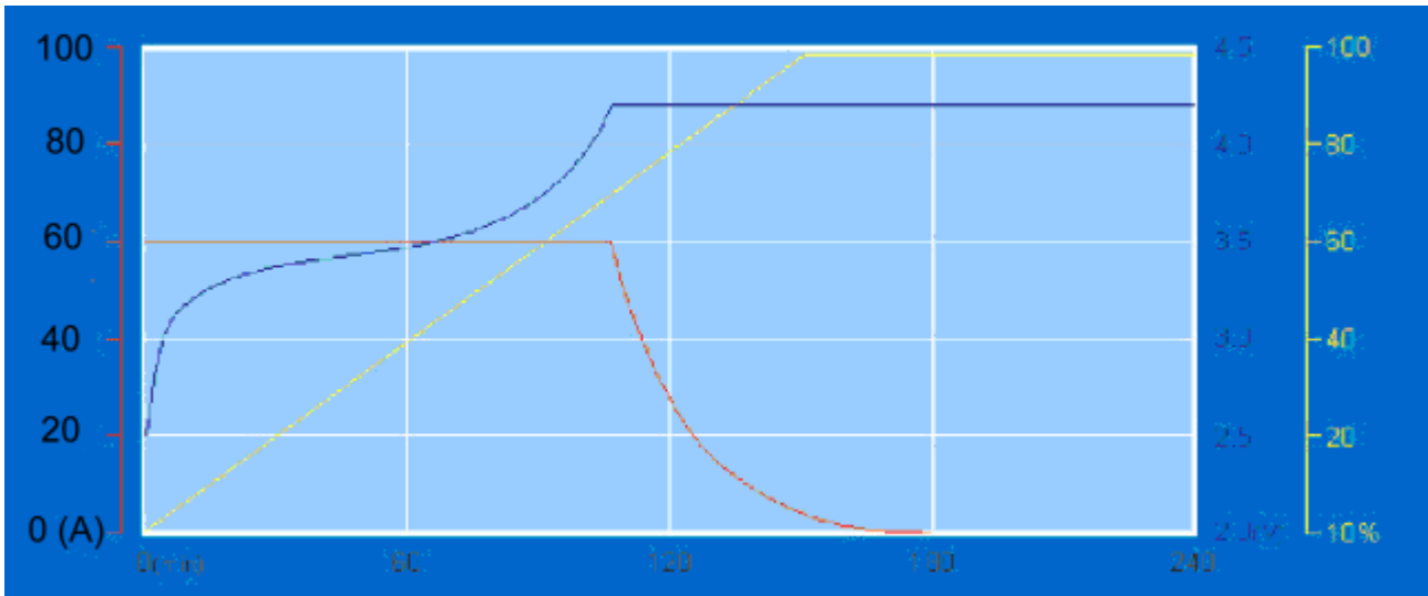
TS-LFP90AHA töltése 25°C környezeti hőmérsékleten Charging at 25°C temperature
