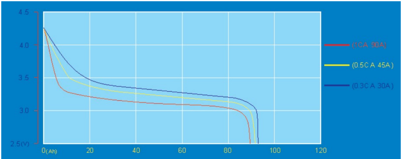
TS-LFP90AHA kisütése 25°C környezeti hőmérsékleten Discharging at 25°C temperature
