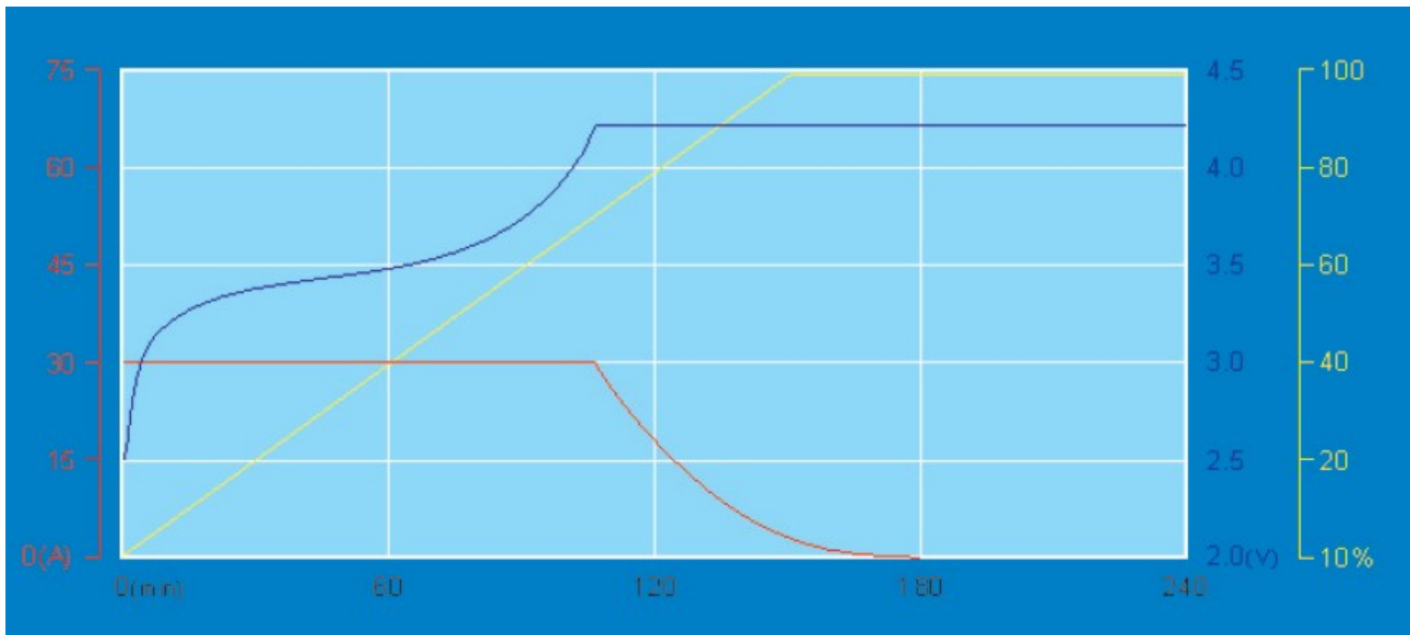
TS-LFP60AHA töltése 25°C környezeti hőmérsékleten Charging at 25°C temperature
