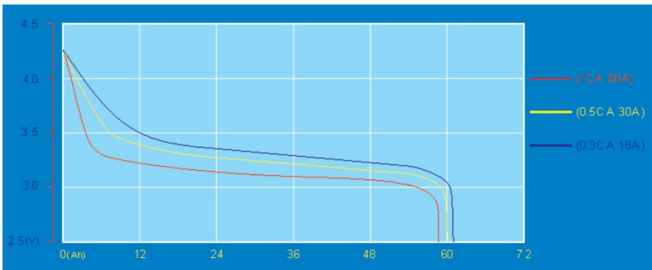
TS-LFP60AHA kisütése 25°C környezeti hőmérsékleten Discharging at 25°C temperature
