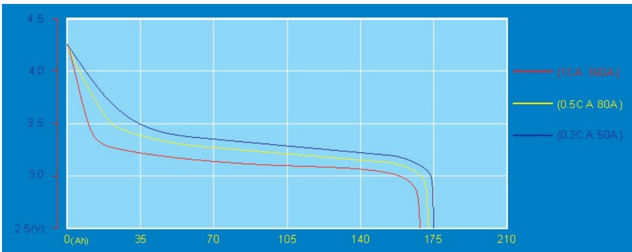
TS-LFP160AHA kisütése 25°C környezeti hőmérsékleten Discharging at 25°C temperature
