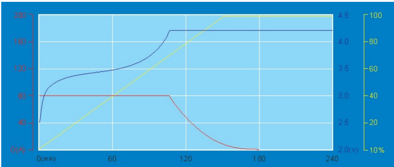
TS-LFP160AHA töltése 25°C környezeti hőmérsékleten Charging at 25°C temperature
